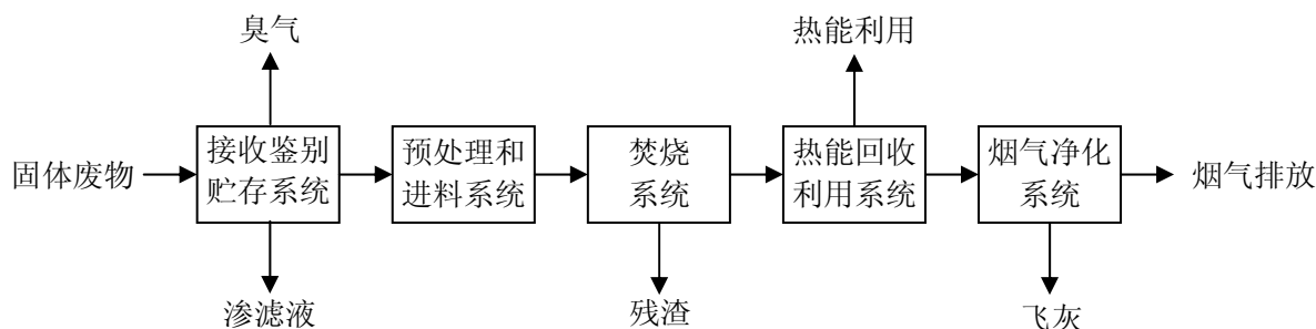
图 3 焚烧工艺流程图
